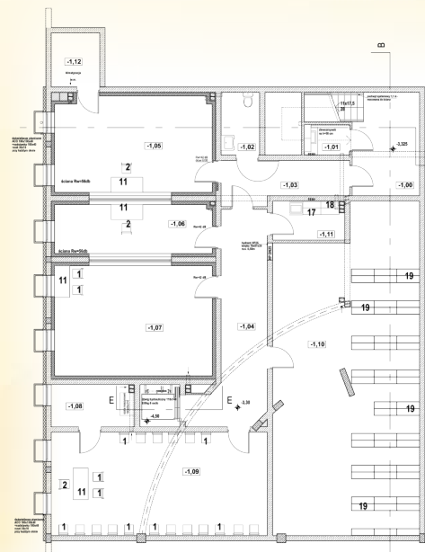
Rzut piwnicy - Centrum Kultury w Witkowie
