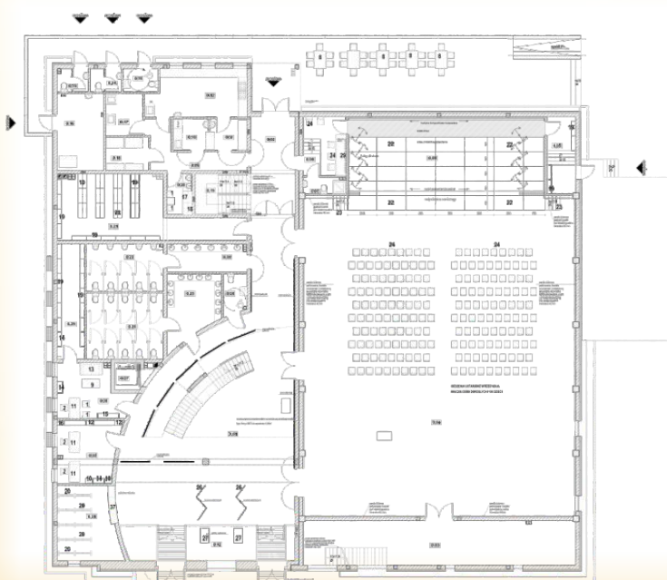
Rzut parteru - Centrum Kultury w Witkowie
